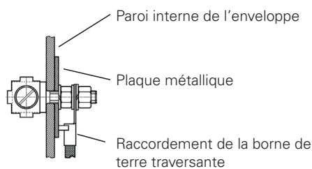
Fig. 5 Borne de terre traversante
